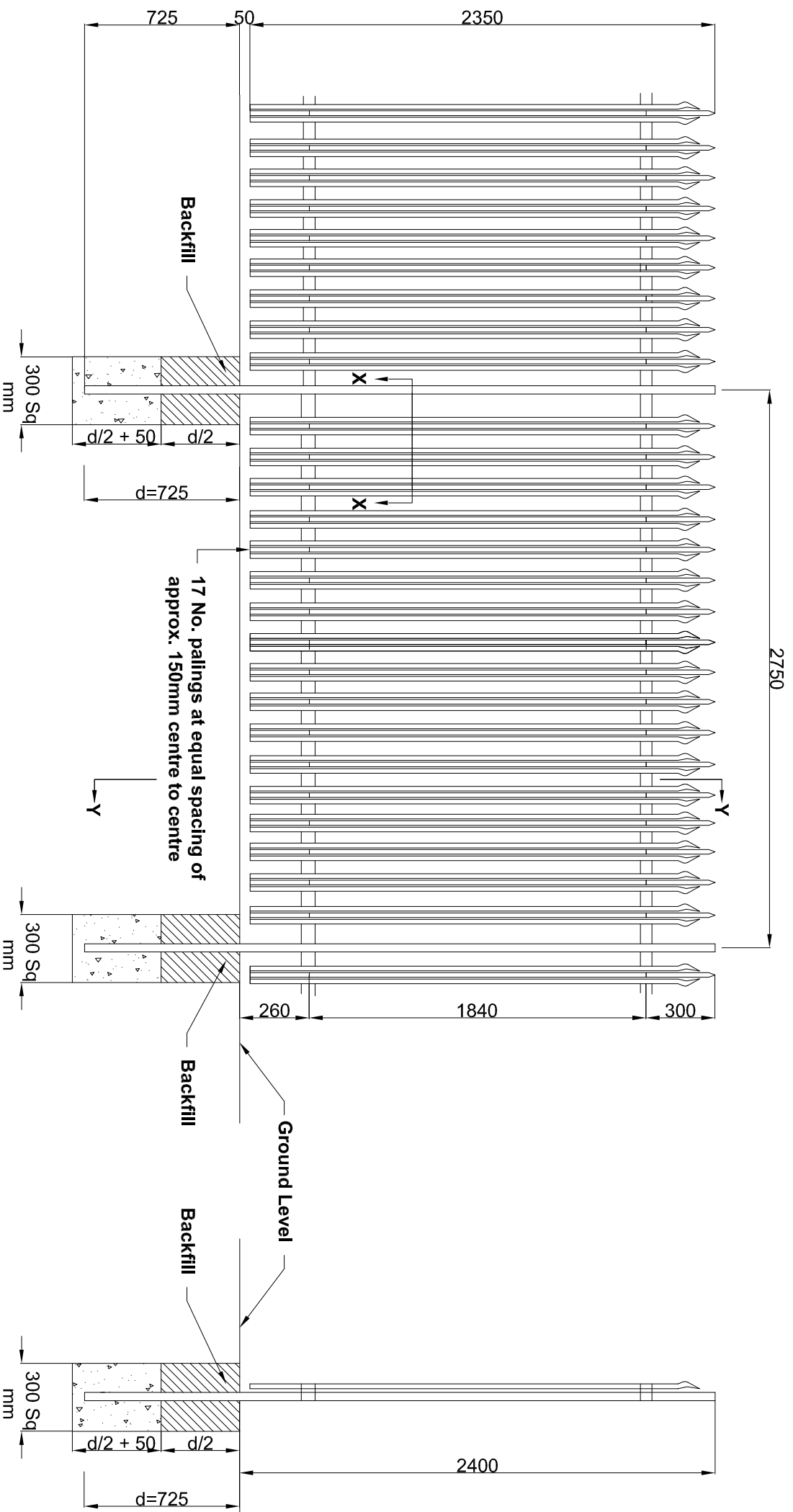
ELEVATION
